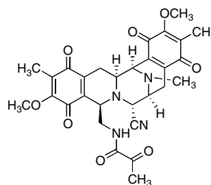
Saframycin A ( 1 )
